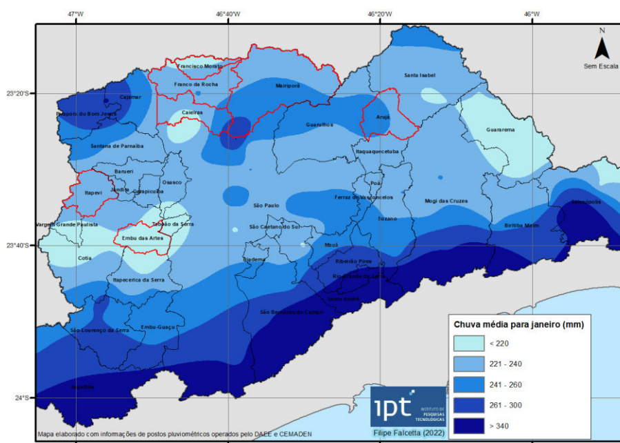
Figura 2 – Chuva média para janeiro na RMSP.
