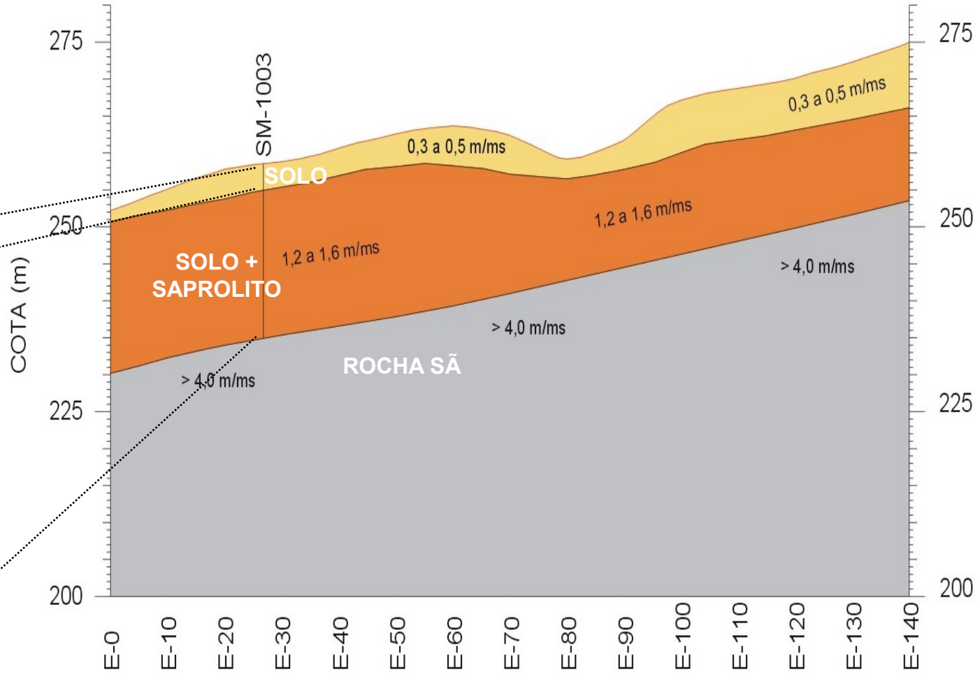
SEÇÃO SÍSMICA INTERPRETADA
