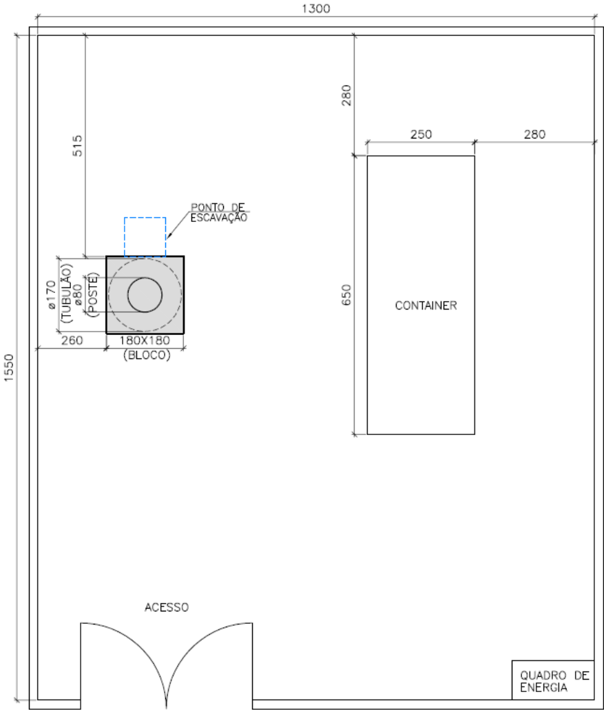
PLANTA DA FUNDAÇÃO
