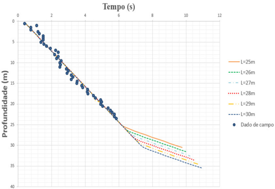
Figura 12. Comparação dos resultados de campo e de simulações, para diferentes comprimentos da estaca.
