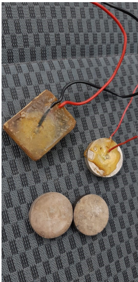
Pastilhas piezoelétricas
