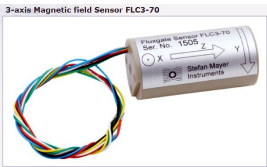
Sensor do magnetômetro fluxgate
