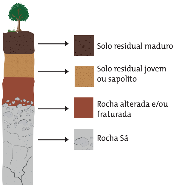
FIGURA 8. Exemplo de um perfil de alteração (manto de alteração) de um terreno.
