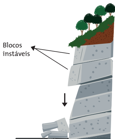
FIGURA 19 – Movimentações com rocha: quedas
