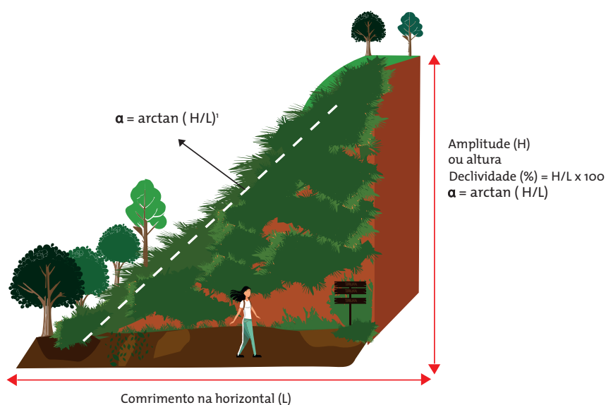
FIGURA 6. Elementos geométricos que proporcionam o cálculo da inclinação e da amplitude de uma encosta e/ou talude.
