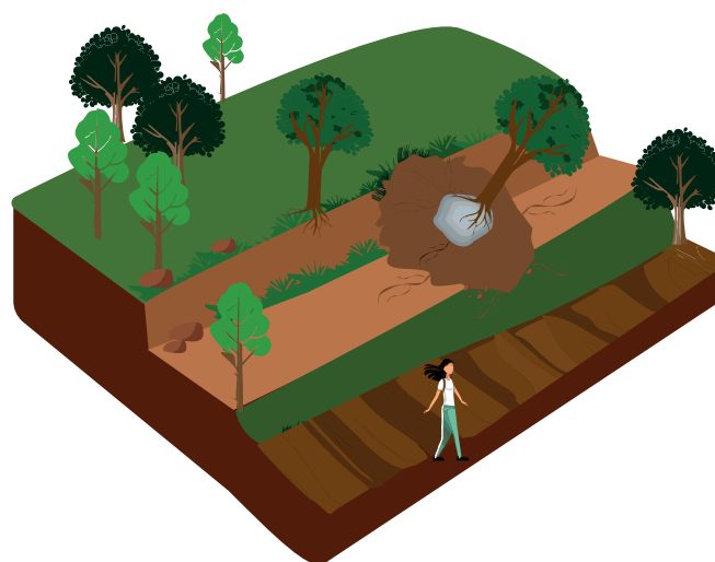
FIGURA 30 – Árvore inclinada decorrente de movimento de massa por ruptura do solo.
