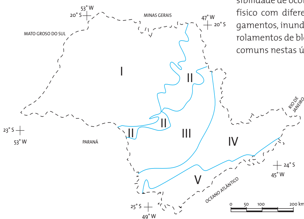
FIGURA 3 : Províncias geomorfológicas.
