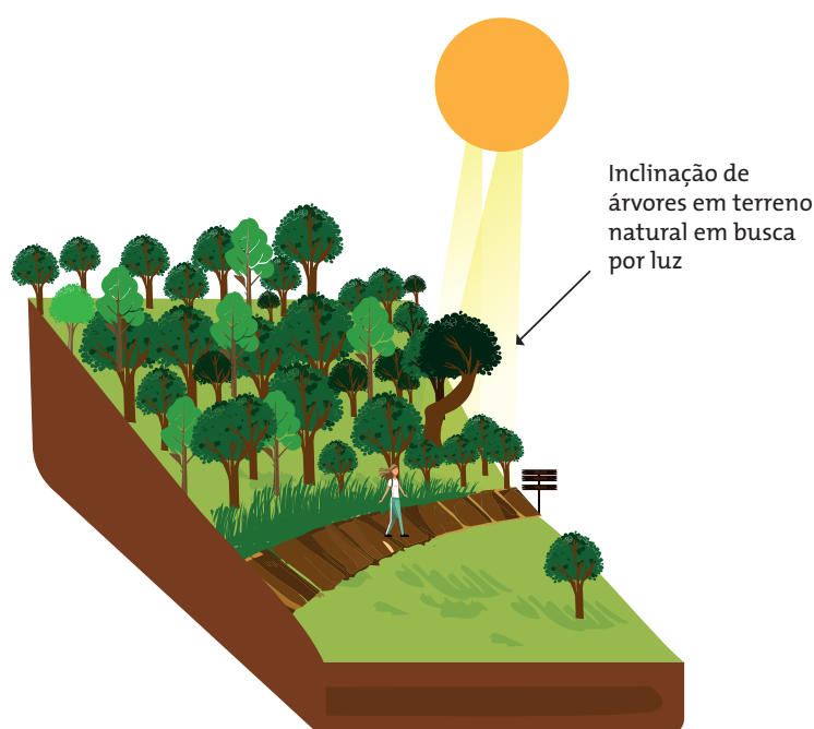
Figura 31 – Fototropismo
