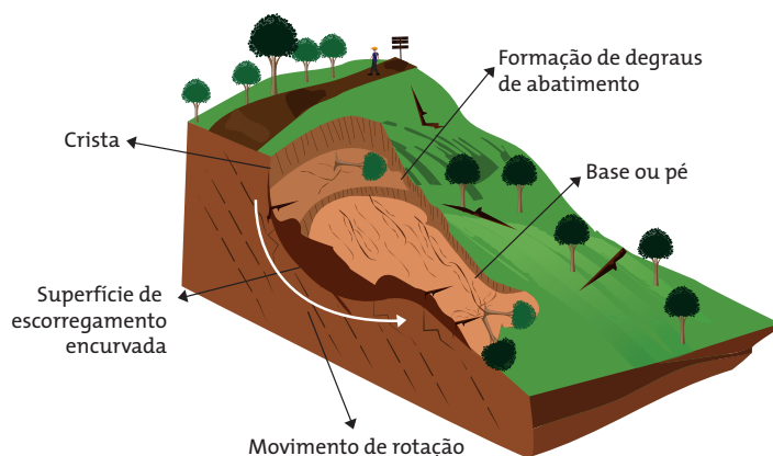
FIGURA 17. Desenho esquemático mostrando um escorregamento circular, também denominado de rotacional.
