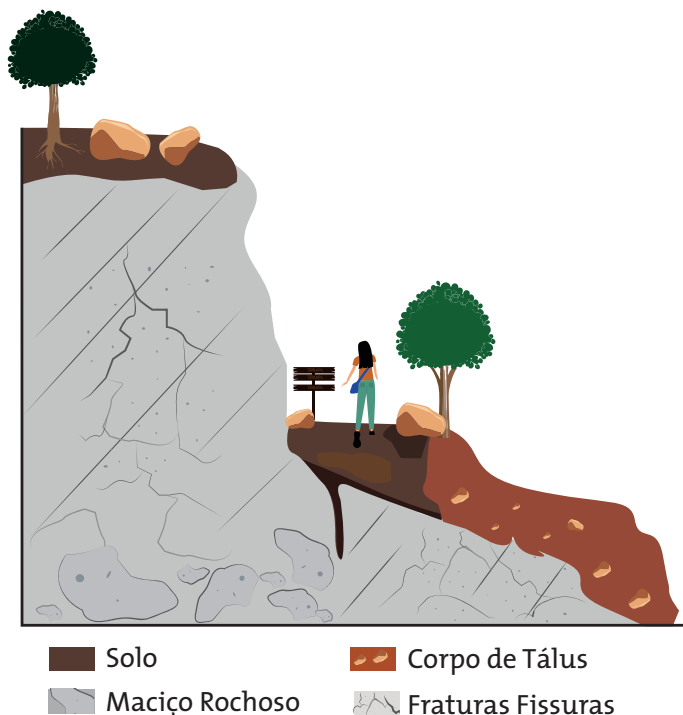
FIGURA 10. Exemplo de formação de paredão rochoso e blocos de rochas dispersos na superfície do terreno.
